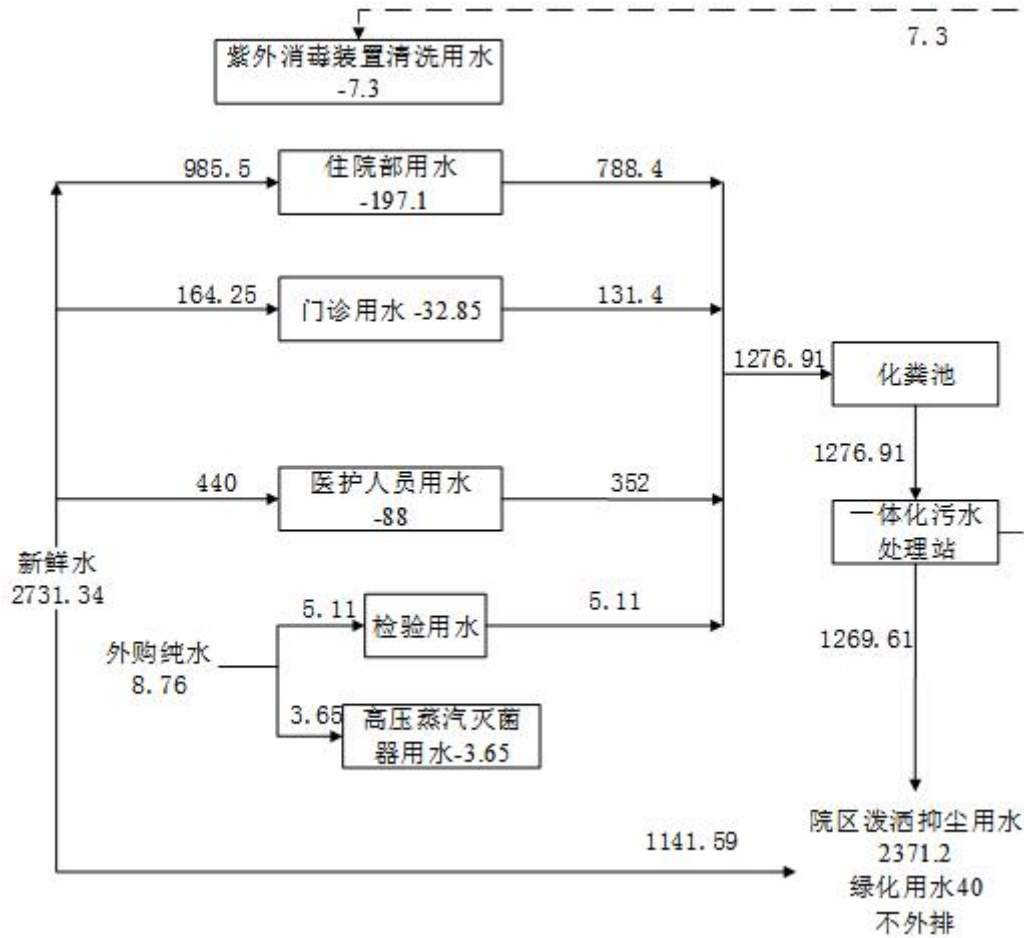
图3.5-1 项目给排水平衡图 单位：m³/a
