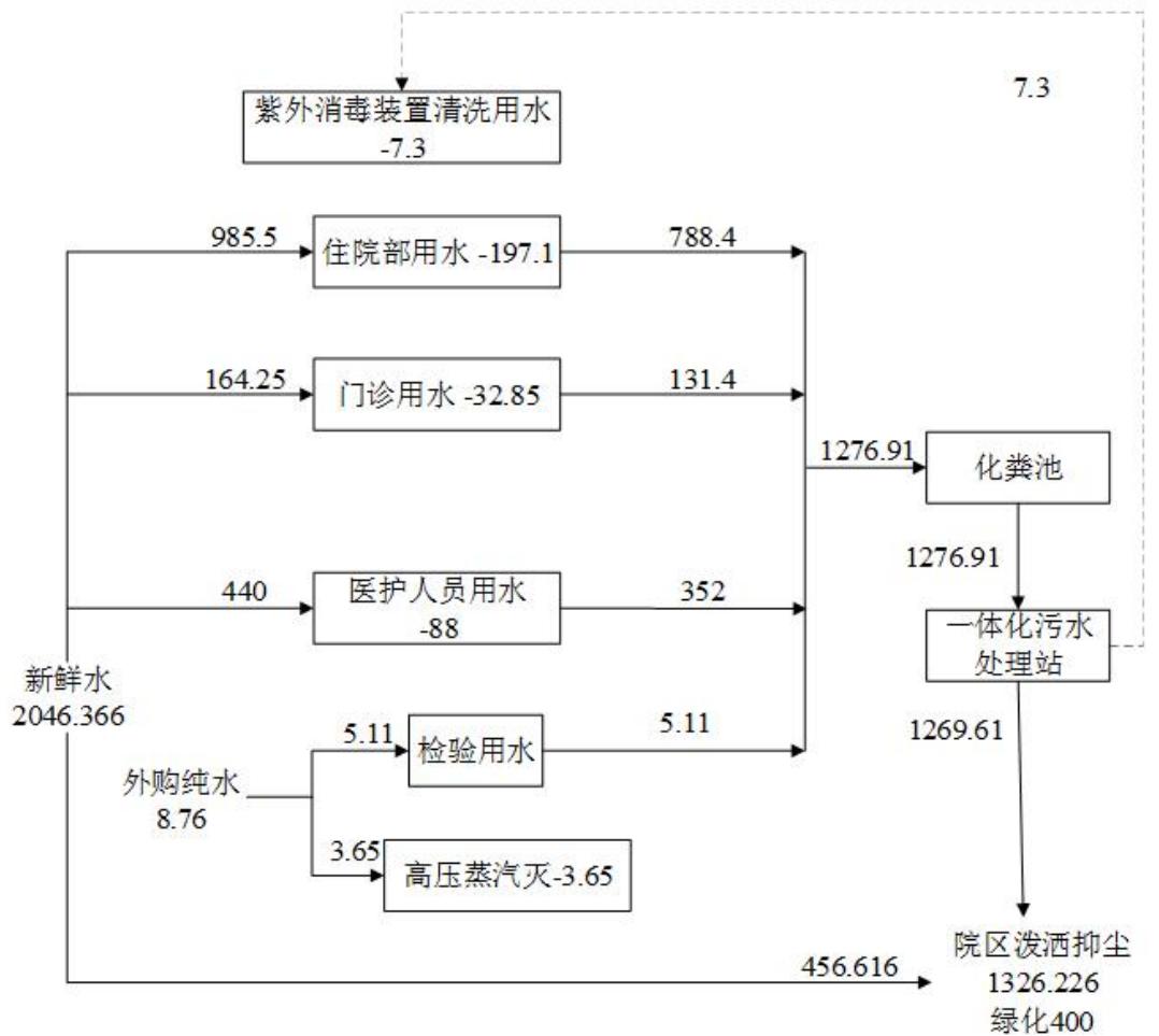
图3.5-1 项目给排水平衡图 单位：m³/a
