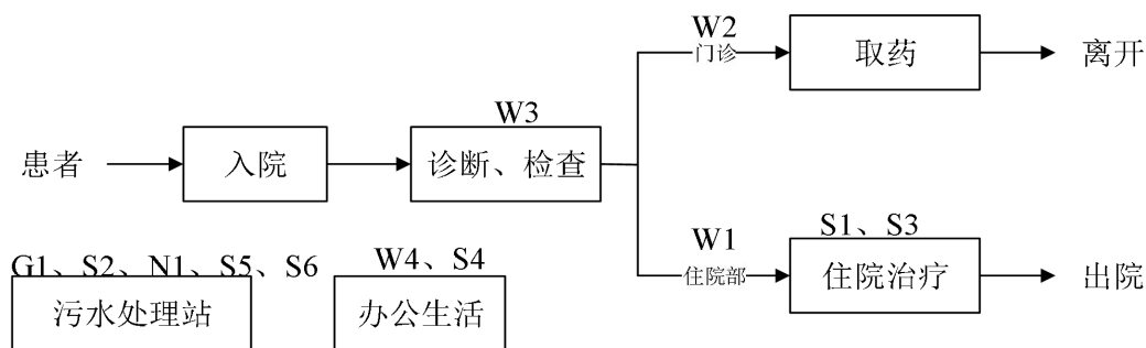
图3.6-1 工艺流程图
