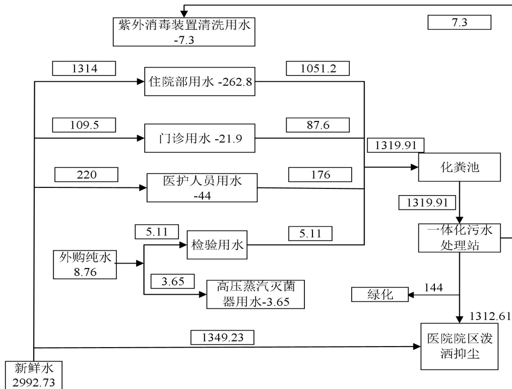
图3.5-1 项目给排水平衡图 单位：m³/a
