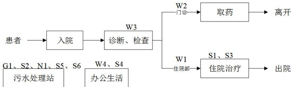
图3.6-1 工艺流程图
