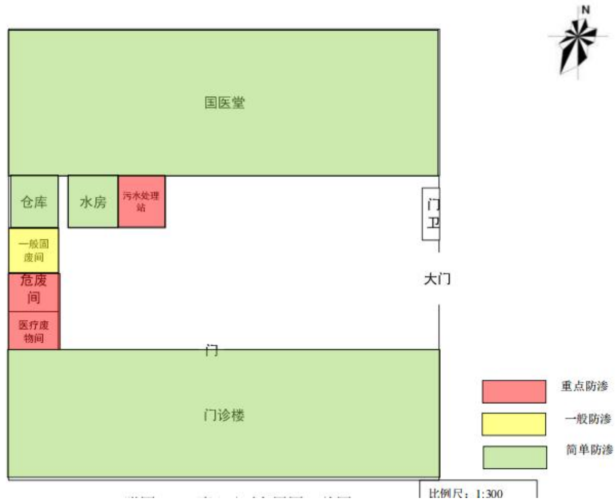
附图3 项目厂区平面布置图 (1: 300)
