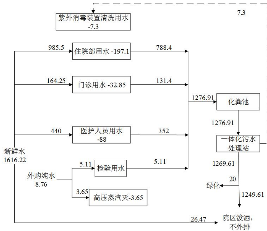
图3.5-1 项目给排水平衡图 单位: m³/a
