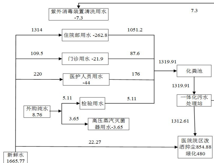
图3.5-1 项目给排水平衡图 单位：m 3 /a
