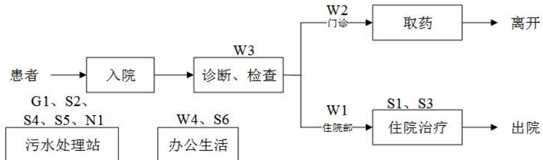
图3.6-1 工艺流程图
